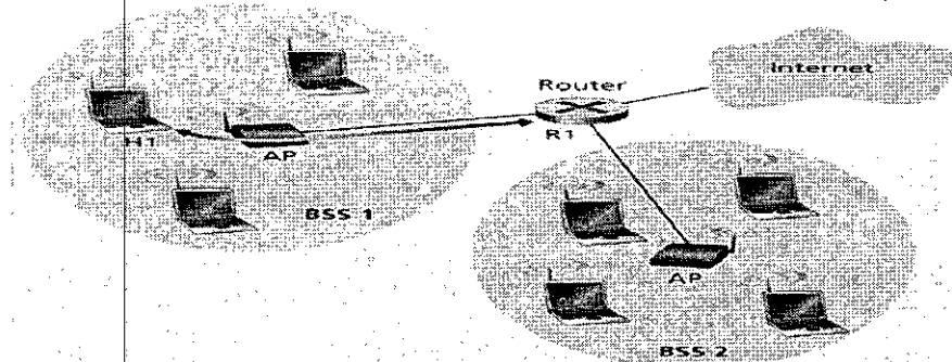
Ilustração de uma conexão de redes IEEE 802.11 com a Internet.
